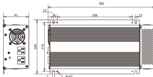
XP1100 寸法:382×195×91mm 重量:4.5kg
