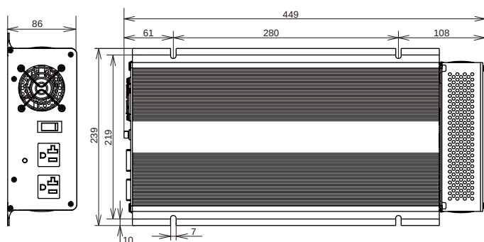
XP2000 寸法:449×239×86mm 重量:6.8kg
