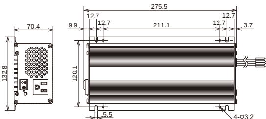
XP250 寸法:275.5×132.8×70.4mm 重量:2.3kg
